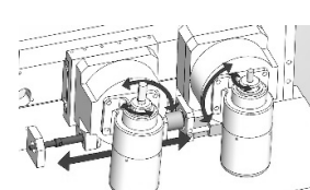
ORIGAMI の外観と内部構成
